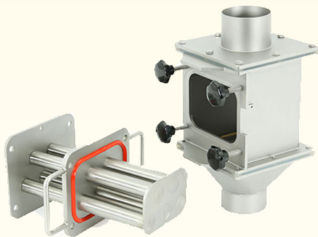
抽屉式除铁器
