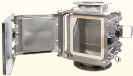
磁板式管道除铁器
